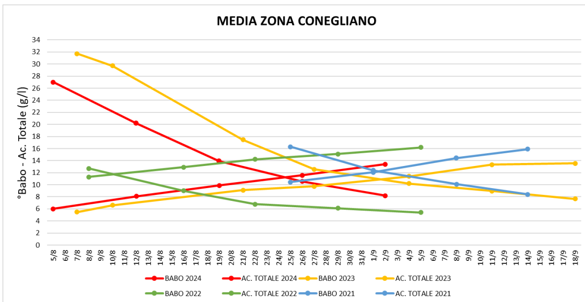
Grafico 1 – Andamento medio della maturazione per la zona di Conegliano.
