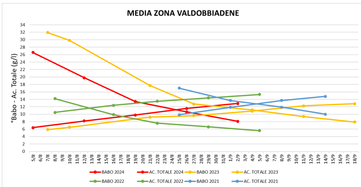
Grafico 2 - Andamento medio della maturazione per la zona di Valdobbiadene.
